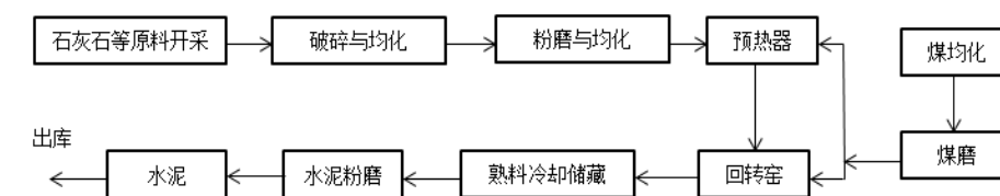
图6 公司水泥生产工艺流程图
