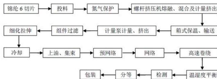
图7 公司锦纶POY生产流程
